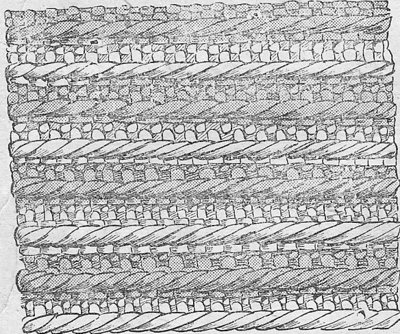
Moitié de la manche.
